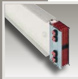
Zucchini railkokersysteem
